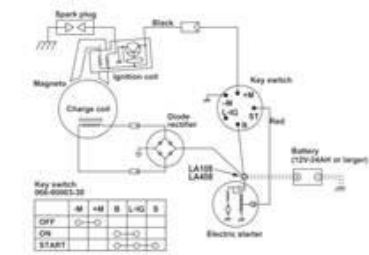
DIAGRAMA DE CABLEADO DL1401EU
