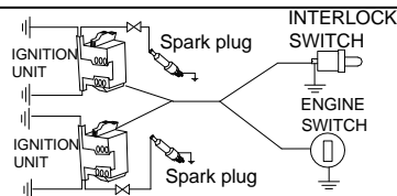
DIAGRAMA DE CABLEADO DL1801VEEU
