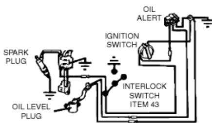
DIAGRAMA DE CABLEADO DL1301EU
